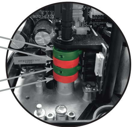
Einstellwerkzeug eingesteckt
